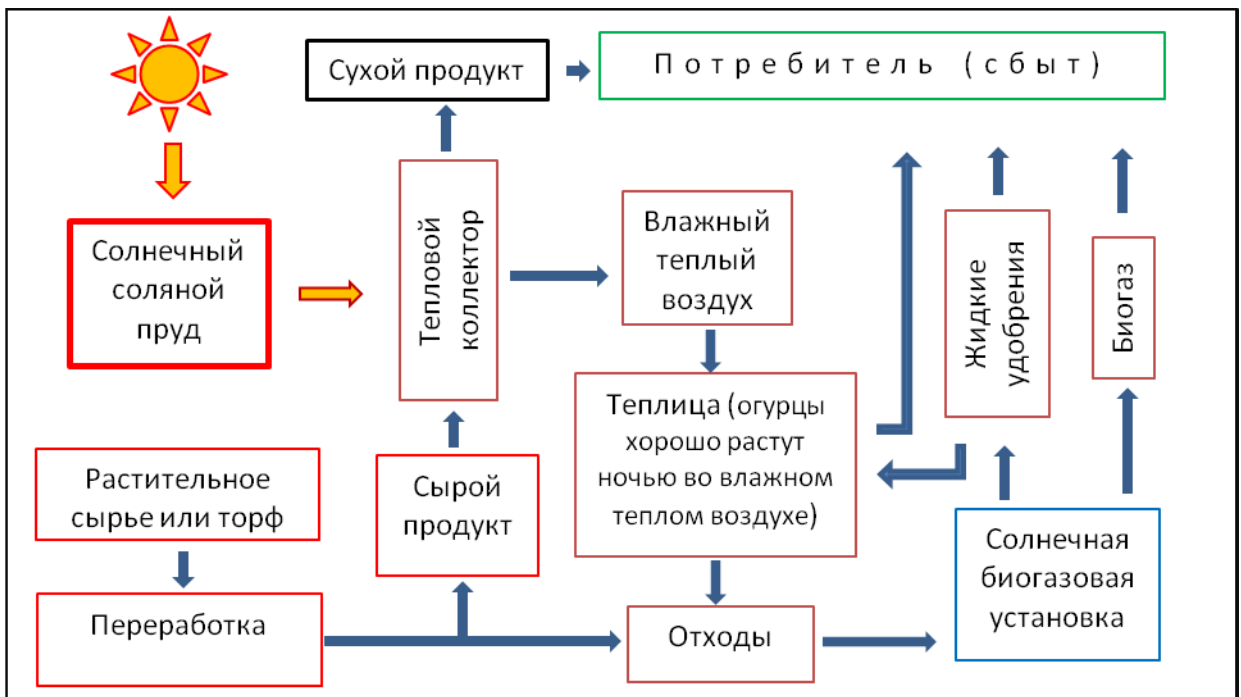
Рисунок 4 – Схема интегрированного комплекса по сушке и производству сельскохозяйственной продукции на базе солнечного соляного пруда
