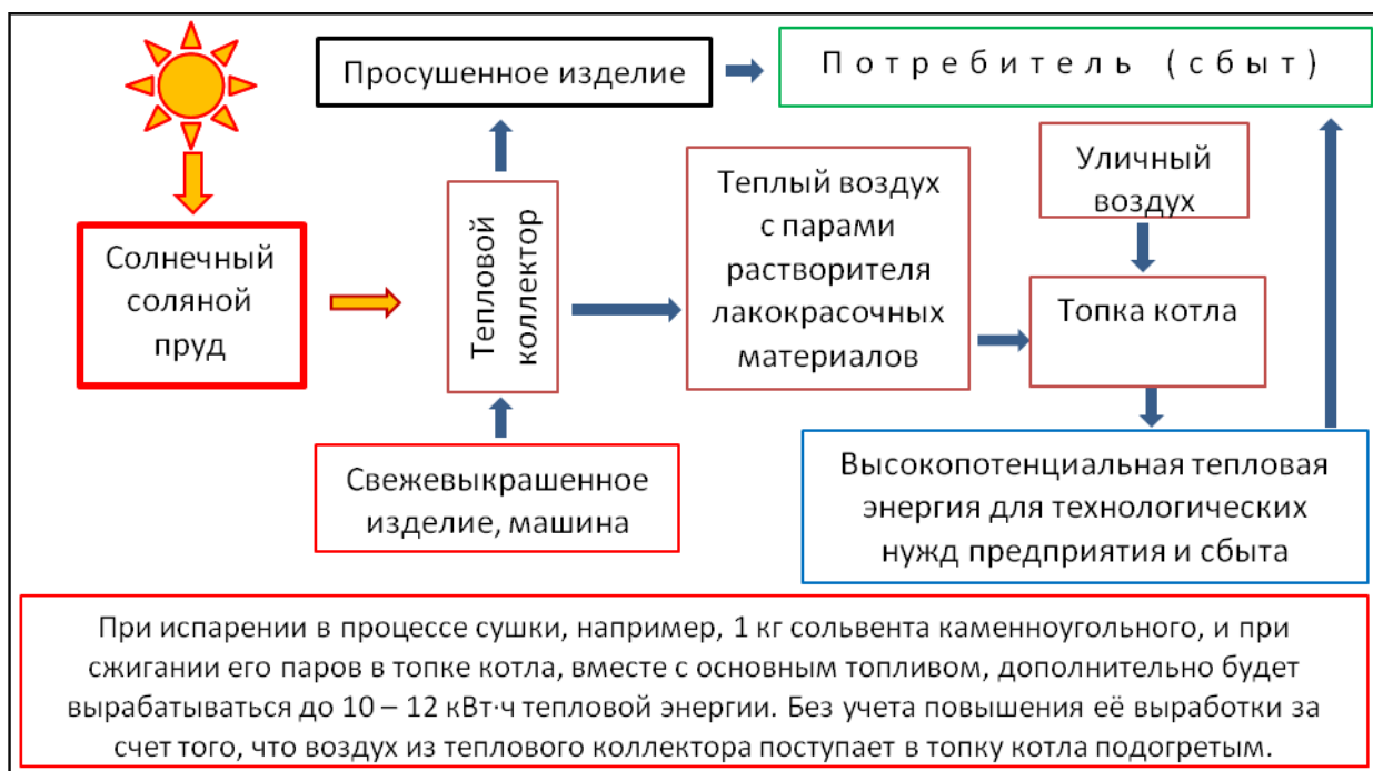
Рисунок 6 – Схема интегрированного участка по сушке изделий после покраски на базе солнечного соляного пруда
