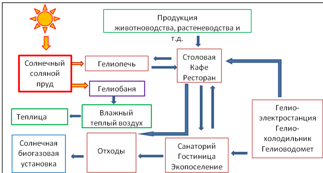
Рисунок 3 – Схема интегрированного комплекса для проживания и отдыха на базе солнечного соляного пруда и котлована со льдом/талой водой
