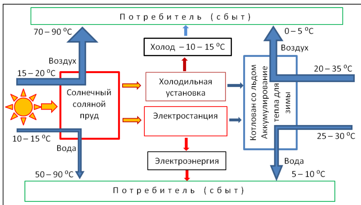
Рисунок 2 – Схема интегрированного комплекса холода, тепло и электроснабжения на базе солнечного соляного пруда и котлована со льдом
